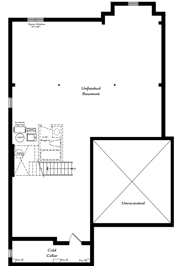
Basement Plan 'A'/'B'
